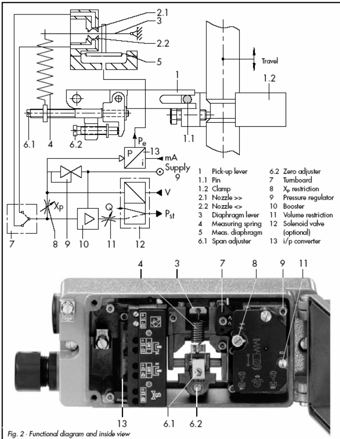
I/P Positioner Type 3767 Samsom Co. : شکل ۴-۴
